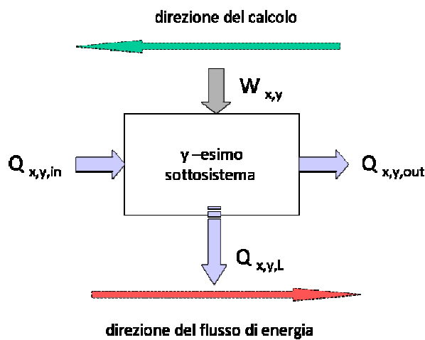
Figura 13- Descrizione funzionale del sottosistema y del sistema impiantistico x
