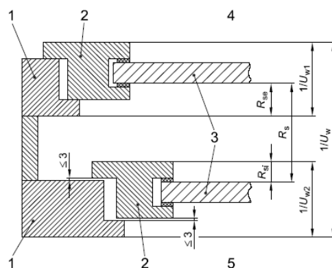
Figura 1 – Esempio di doppio serramento
