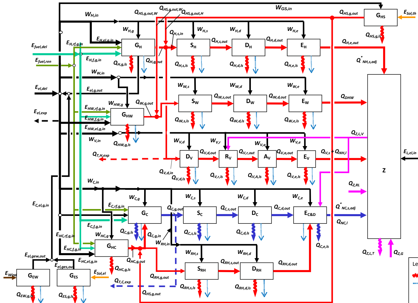
Figura 12 – Schematizzazione dell'impianto termico con generazione termica separata
