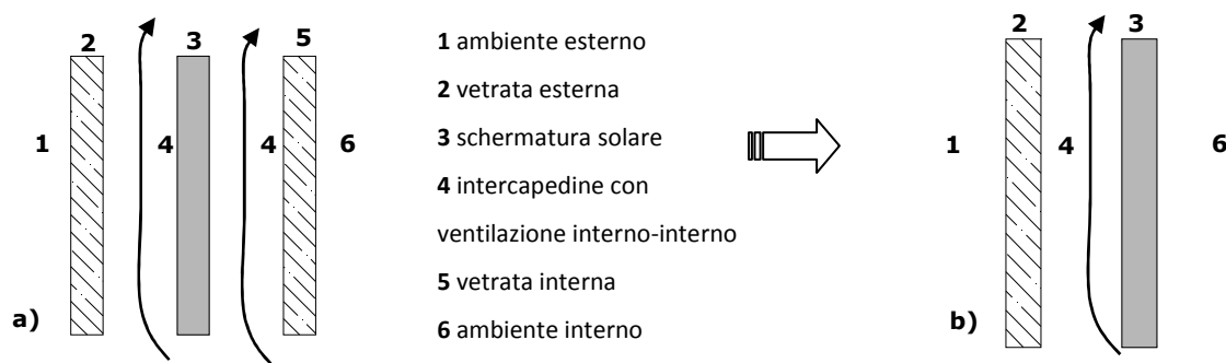
Figura 9 – Schematizzazione di una schermatura solare integrata con intercapedine ventilata interno su interno e del suo sistema equivalente ai fini del calcolo semplificato del fabbisogno estivo
