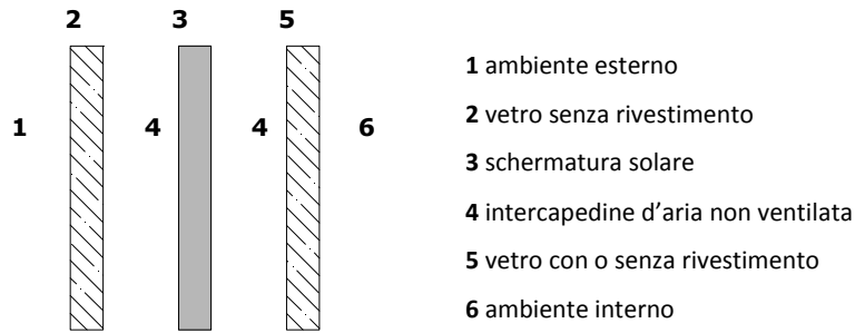
Figura 7 – Schematizzazione di una schermatura solare integrata con intercapedine non ventilata
